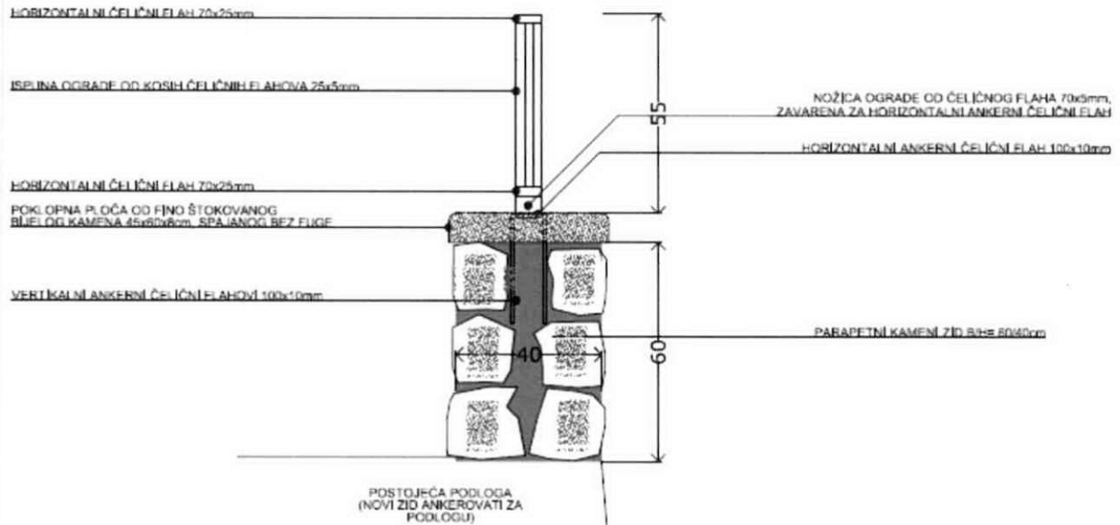
Detalj zida
